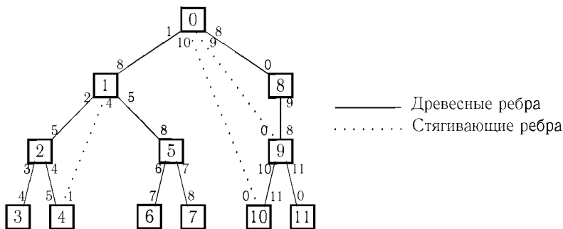
Рис. 4.15. Схема интервальной разметки в глубину
