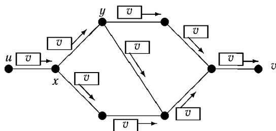
Рис. 4.3. Пример разветвляемой маршрутизации
