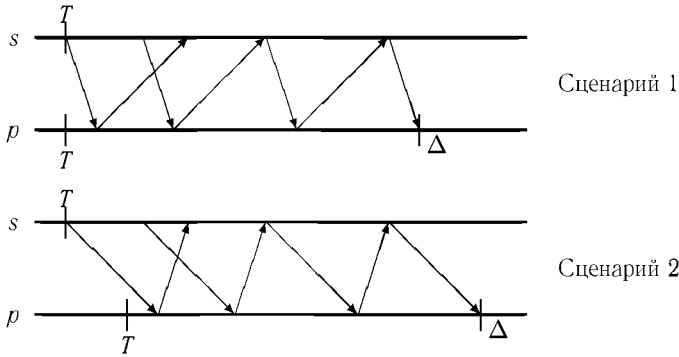
Рис. 15.5. Сценарии работы детерминированного протокола
