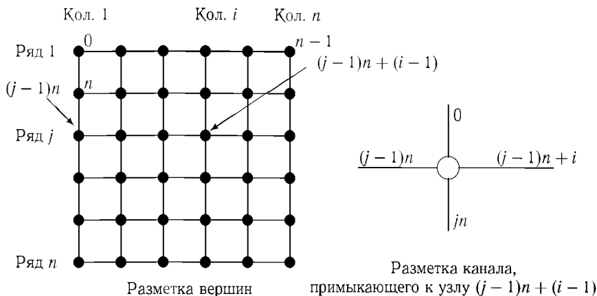
Рис. 4.19. Оптимальная ILS для решетки размера n \times n
