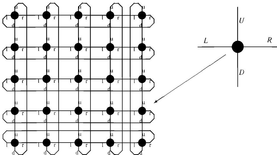
Рис. Б.8. Восприятие направления в торе
