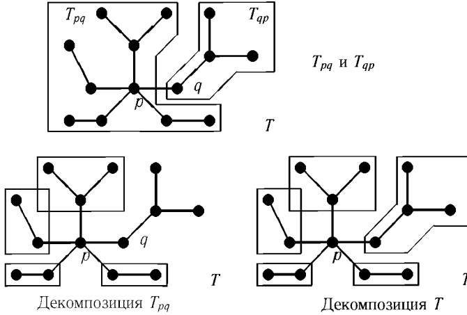
Рис. 6.3. Поддеревья T_{pq}
