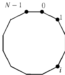
Рис. 7.4. Наихудший возможный сценарий для алгоритма Ченя—Робертса
