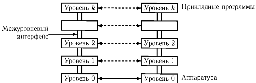
Рис. 1.4. Многоуровневая архитектура сети
