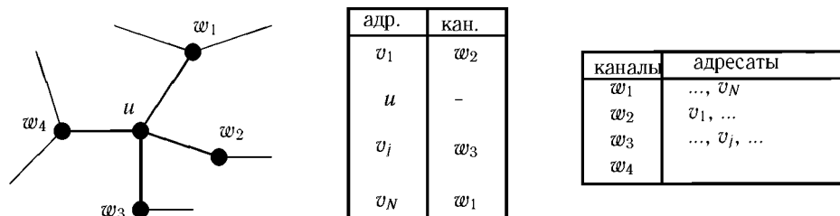
Рис. 4.11. Сокращение размера таблиц маршрутизации
