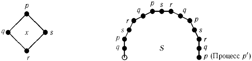
Рис. 9.2. Построение неправильного вычисления
