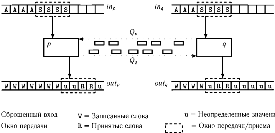
Рис. 3.2. Протокол раздвижного окна
