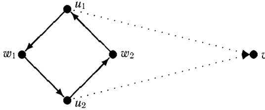
Рис. 5.2. Маршрутизация, недопустимая для контроллера dest
