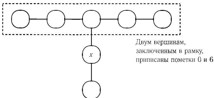
Рис. 4.17. Граф с тремя отростками
