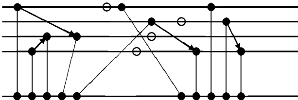
Рис. 10.3. Выполнение F
