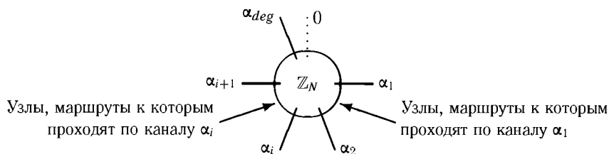
Рис. 4.14. Разбиение множества \mathbb{Z}_N в узле
