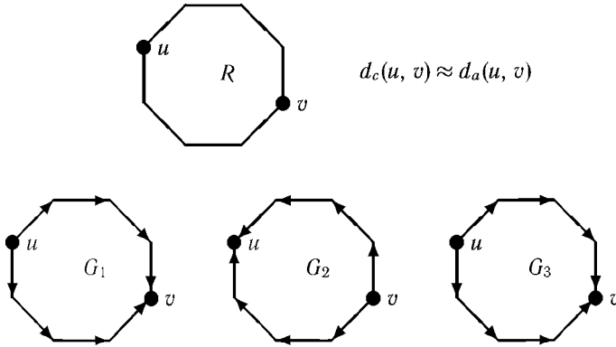
Рис. 5.4. Ациклическое ориентированное покрытие для кольца
